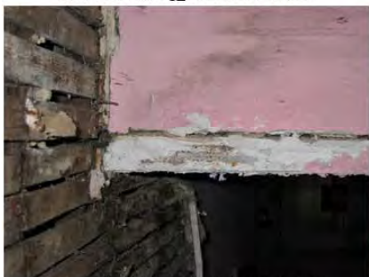
Room 103-Ceiling_10-2007-02-02.JPG
